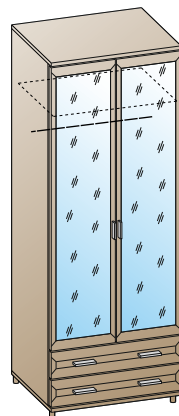
ШК-2807 2264x900x576
